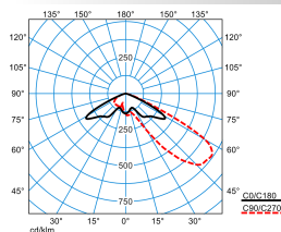
LnPlus 40-AM19L-SLR3/5100-740 6G1 ET (CLO initial value)
