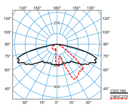
Publisca P1W-AB2L-LR/1500-740 2G1S ET (CLO end value)
