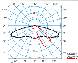
Publisca P1W-AB2L-LR/1500-740 2G1S ET (CLO initial value)
