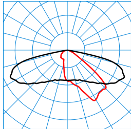
LIQ 50N-AB2L-LR/3500-727 4G1 ET (CLO end value) TX777778 ■ C0 - C180 ■ C90 - C270 DIN 5040: A30 UTE: 1,00 G DLOR: 100 % ULOR: 0 % CEN Flux Code: 34 71 96 100 100 0 0 0 0
