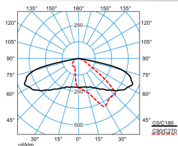
LIQ 50N-AB2L-LR/3500-727 4G1 ET (CLO end value) TX777778
