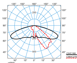
Publisca P2-AB2L-LRA/4200-730 6G1S ET (CLO initial value) TX301953 DIN 5040: A30 UTE: 1,00 G DLOR: 100 % ULOR: 0 % CEN Flux Code: 35 74 97 100 100
