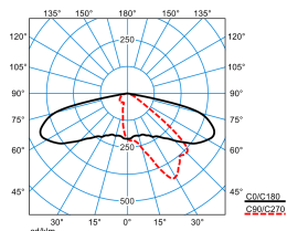
Publisca P3-AB2L-LRA/4200-740 4G1
