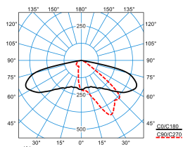
Publisca P3-AB2L-LRA/4200-740 4G1 ET (CLO end value)
