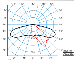
Publisca P3-AB2L-LRA/4200-740 4G1 ET (CLO initial value)
