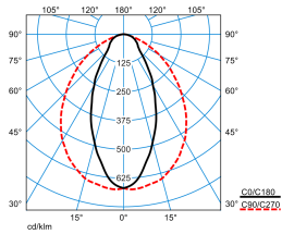
Nextrema G3 TB 8000-840 ET +LV TX770423
