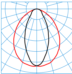
Nextrema G3 TB 8000-840 ET +LV TX770423
