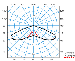
Publisca P1-RB6L-LRA/1000-730 2G1S ET (CLO initial value) TX301674
