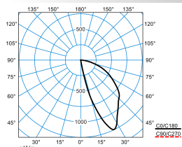
Linell 3PID5 WW-D-R 10-927 ETDD 05
