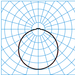
Olisq QWD3 DW 45-840 ETBLE +DMR IP54 IK + Olisq QWD3 ZDR 1/2 01 TX461779 ■ C0 - C180 ■ C90 - C270
