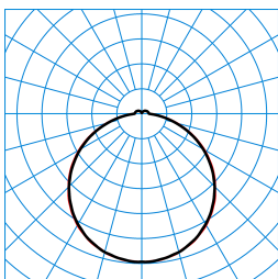
Olisq QWD3 DW 45-840 ETBLE +DMR IP54 IK + Olisq QWD3 ZDR 1/2 05 TX461797 ■ C0 - C180 ■ C90 - C270
