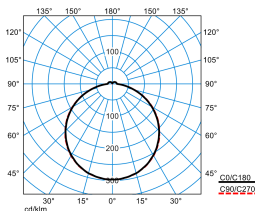
Olisq QWD3 DW 45-840 ETBLE +DMR IP54 IK + Olisq QWD3 ZDR 1/2 05
