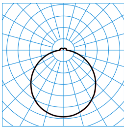
Olisq QWD3 DW 45-840 ETBLE +DMR IP54 IK TX778397 ■ C0 - C180 ■ C90 - C270
