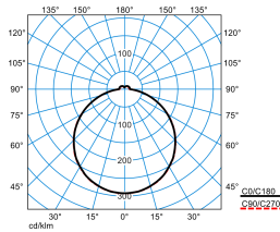
Olisq QWD3 DW 45-840 ETBLE +DMR IP54 IK
