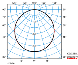
Olisq QWD3 DW 45-840 ETBLE +DMR IP54 IK + Olisq QWD3 ZDR 1/1 01
