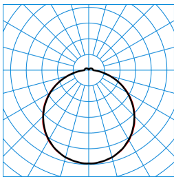
Olisq QWD3 DW 45-840 ETBLE +DMR IP54 IK + Olisq QWD3 ZDR 1/2 03 TX461297 ■ C0 - C180 ■ C90 - C270
