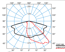
Cuvia 60-AB6L-LR/4200-740 8G1S ET
