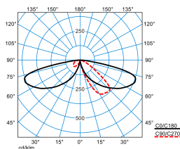
LTX LT-AB2L-LRA/15/18/26-730 4G1 (1800 lm)
