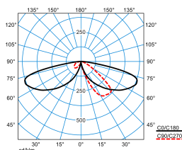
LTX LT-AB2L-LRA/15/18/26-730 4G1 (2600 lm)
