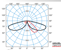
LTX LT-AB2L-LRA/15/18/26-730 4G1 (1500 lm)
