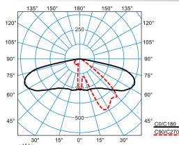
Publisca P1-AB2L-LRA/1500-740 2G1S TX047549 DIN 5040: A30 UTE: 1,00 G DLOR: 100 % ULOR: 0 % CEN Flux Code: 34 70 96 100 100
