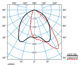
Jovie 70-AM3L-8-100-740-CLO-E
