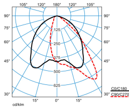
Jovie 70-AM3L-8-100-740-CLO-B
