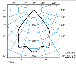
LPCV 3P2 L-W19 05 65-830 K03 ET 05
