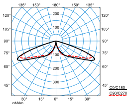
CS 19 100-RB6L-LRA/2900-730 2G1S ET (CLO initial value)
