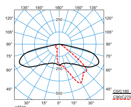
Publisca P3-AB2L-LRA/2200-740 4G1
