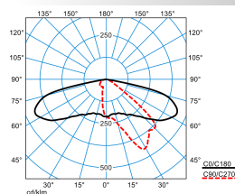
Publisca P3-AB2L-LRA/2200-740 4G1 ET (CLO initial value)
