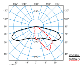
Publisca P3-AB2L-LRA/2200-740 4G1 ET (CLO end value)
