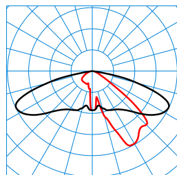
Publisca P2-AB2L/4600-740 6G1S ETDD (CLO end value) TX301524 ■ C0 - C180 ■ C90 - C270 DIN 5040: A30 UTE: 1,00 G DLOR: 100 % ULOR: 0 % CEN Flux Code: 35 74 97 100 100
