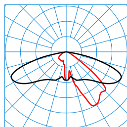
Publisca P2-AB2L/4600-740 6G1S ETDD (CLO initial value) TX301580 ■ C0 - C180 ■ C90 - C270 DIN 5040: A30 UTE: 1,00 G DLOR: 100 % ULOR: 0 % CEN Flux Code: 35 74 97 100 100
