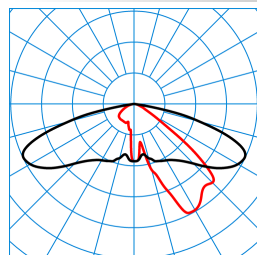
Publisca P2-AB2L/4600-740 6G1S TX047727 ■ C0 - C180 ■ C90 - C270 DIN 5040: A30 UTE: 1,00 G DLOR: 100 % ULOR: 0 % CEN Flux Code: 35 74 97 100 100
