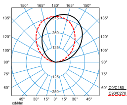
Sanesca W2 5000 ETDD8/ET 840 01 (DCW) (room light) TX874748
