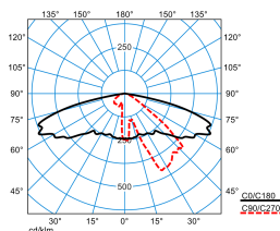
Publisca P1W-AB2L-LRA/1800-730 2G1S ET (CLO end value)
