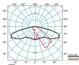
Publisca P1W-AB2L-LRA/1800-730 2G1S ET (CLO initial value)
