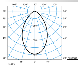
Ambiella G2 C07 HR LED2000-830 ET 01
