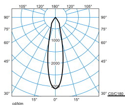
E-Line PRO 78 BV G2 RF-MF 40-840 M35 ET 01 01
