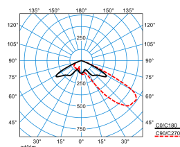
LnPlus 40-AM19L-SLR2/3200-722 4G1 ET (CLO end value)
