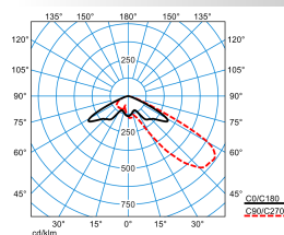
LnPlus 40-AM19L-SLR2/3200-722 4G1 ET (CLO initial value)
