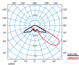
LnPlus 70-AM19L-SLR2/51000-722 48G1 ET (CLO initial value)
