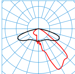
Publisca P1-AB2L-LR/3200-740 4G1S TX047528 ■ C0 - C180 ■ C90 - C270 DIN 5040: A30 UTE: 1,00 G DLOR: 100 % ULOR: 0 % CEN Flux Code: 35 73 97 100 100
