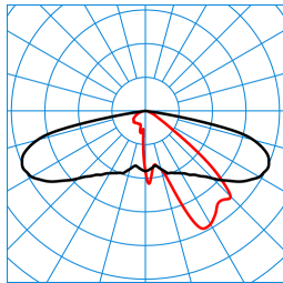
Publisca P2-AB2L/2600-740 3G1S TX047715 ■ C0 - C180 ■ C90 - C270 DIN 5040: A30 UTE: 1,00 l DLOR: 100 % ULOR: 0 % CEN Flux Code: 34 71 96 100 100
