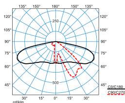
Publisca P1-AB2L/1800-740 2G1S ETDD (CLO initial value)
