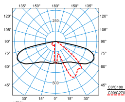
Publisca P1-AB2L/1800-740 2G1S ETDD (CLO end value)
