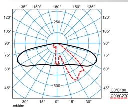
Publisca P1-AB2L/1800-740 2G1S
