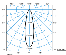
E-Line PRO 78 BV G2 RF-MF 20-M M52 ET 05 Blank
