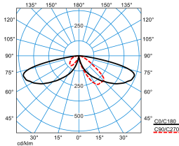
LTX ZT-AB2L-LR/1800-740 2G1 ET
