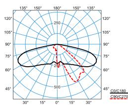
Publisca P1-AB2L-LRA/2000-730 3G1S ET (CLO end value)
