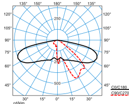
Publisca P1-AB2L-LRA/2000-730 3G1S TX047554 DIN 5040: A30 UTE: 1,00 l DLOR: 100 % ULOR: 0 % CEN Flux Code: 34 71 96 100 100
