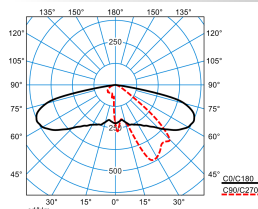
Publisca P1-AB2L-LRA/2000-730 3G1S ET (CLO initial value)
