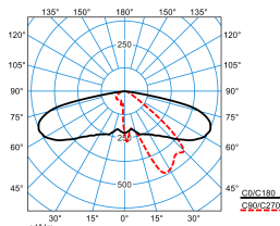
Publisca P1-AB2L-LRA/2000-730 3G1S ET (CLO initial value) TX301112 DIN 5040: A30 UTE: 1,00 l DLOR: 100 % ULOR: 0 % CEN Flux Code: 34 71 96 100 100
