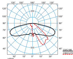
Publisca P1-AB2L-LRA/2000-730 3G1S ET (CLO end value) TX301417 DIN 5040: A30 UTE: 1,00 l DLOR: 100 % ULOR: 0 % CEN Flux Code: 34 71 96 100 100
