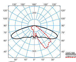
Publisca P1-AB2L/5600-740 6G1S
