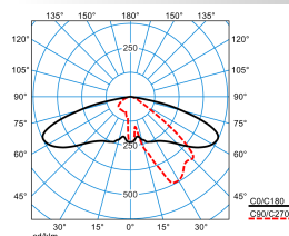
Publisca P1-AB2L/5600-740 6G1S ETDD (CLO initial value)
