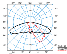
Publisca P1-AB2L/5600-740 6G1S ETDD (CLO end value)
