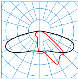
Jovie 50-AB2L-ML-LR/4600-6800-730 6G1 ET (CLO end value) TX271467
