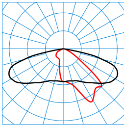
Jovie 50-AB2L-ML-LR/4600-6800-730 6G1 ET (CLO initial value) TX271464
