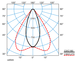
E-Line PRO 78IP50 MironaF HR 270-840 ETDD L225 01 01 (LEO2)
