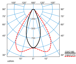
E-Line PRO 78IP50 MironaF HR 270-840 ETDD L225 01 01 (LEO3)
