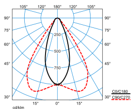
E-Line PRO 78IP50 MironaF HR 270-840 ETDD L150 01 01 IP50 (LEO1)
