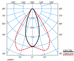
E-Line PRO 78IP50 MironaF HR 270-840 ETDD L150 01 01 IP50 (LEO2)
