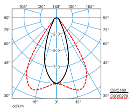
E-Line PRO 78IP50 MironaF HR 270-840 ETDD L225 01 01 (LEO1)
