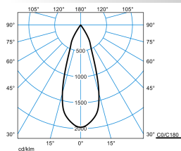
CPL G2 3P FL 30-EW M48 ETDD L1,5 01
