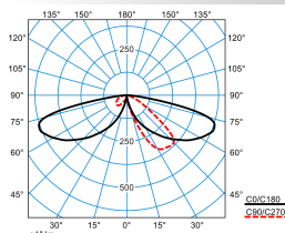
LTX KT-AB2L-LRA/15/18/26-740 4G1 (1500 lm)
