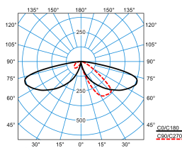
LTX KT-AB2L-LRA/15/18/26-740 4G1 (2600 lm)
