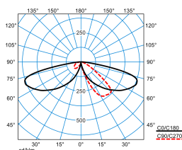
LTX KT-AB2L-LRA/15/18/26-740 4G1 (1800 lm)
