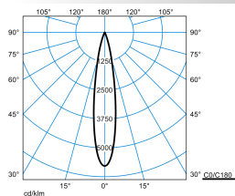
Ly G2 3PID-ST L-SP 01 20-830 M25 ETDD 01
