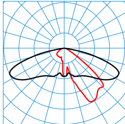
Publisca P1-AB2L-LRA/5600-740 6G1S TX047576 ■ C0 - C180 ■ C90 - C270 DIN 5040: A30 UTE: 1,00 G DLOR: 100 % ULOR: 0 % CEN Flux Code: 35 74 97 100 100
