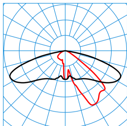
Publisca P1-AB2L-LRA/5600-740 6G1S ET (CLO initial value) TX300594 ■ C0 - C180 ■ C90 - C270 DIN 5040: A30 UTE: 1,00 G DLOR: 100 % ULOR: 0 % CEN Flux Code: 35 74 97 100 100
