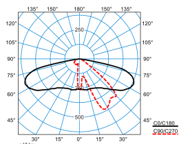
Publisca P1-AB2L-LRA/1100-740 2G1S ET (CLO end value)
