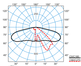
Publisca P1-AB2L-LRA/1100-740 2G1S ET (CLO initial value)
