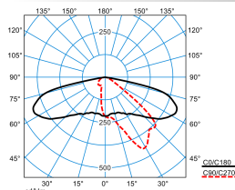
Cuvia 60-AB2L-LR/5600-740 8G1S ET
