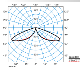
LTX KT-RB6L-LRA/15/18/26-740 4G1 (1500 lm)
