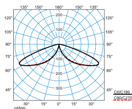
LTX KT-RB6L-LRA/15/18/26-740 4G1 (2600 lm)
