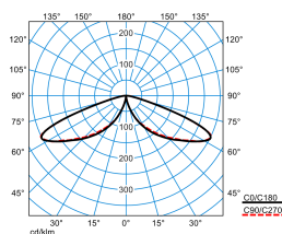
LTX KT-RB6L-LRA/15/18/26-740 4G1 (1800 lm)
