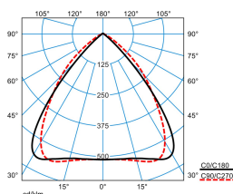
ELINE HE LN60-160 ML 830 L225 2 20
