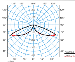
LTX L-RB6L-LRA/3800-730 4G1 ETDD
