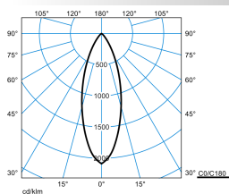
Amatris RC1 SRRFL 4-9MC ET 05 2KIT + HC-19 05 (stage 1)
