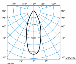
Amatris RC1 SRRFL 4-9MC ET 05 2KIT + PC IP54 (stage 1)
