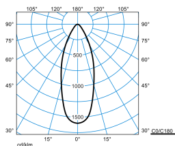
Amatris RC1 SRRFL 4-9MC ET 05 2KIT + PC IP54 (stage 2)
