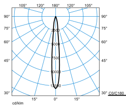
Altigo G2 30 RE1L/1000-830 1G1P + VE IP66 24V DC 60W
