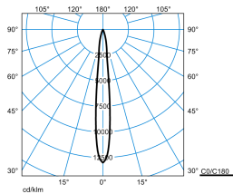
Altigo G2 30 RE1L/1000-830 1G1P + VE IP66 24V DC 250W
