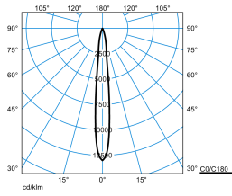
Altigo G2 30 RE1L/1000-830 1G1P + VE IP66 24V DC 130W
