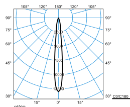
Altigo G2 30 RE1L/1000-830 1G1P + VE IP66 24V DC 80W
