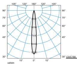
Altigo G2 30 RE1L/1000-830 1G1P + VE IP66 24V DC 80W
