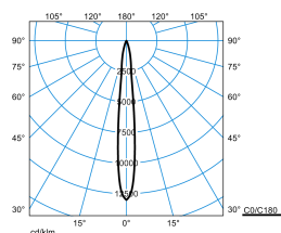
Altigo G2 30 RE1L/1000-830 1G1P + VE IP66 24V DC 130W
