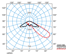
LnPlus 40-AM19L-LR/5100-730 6G1 ET (CLO initial value)
