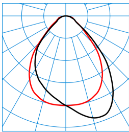
ArmoFit G2 D3 P-WW 53-840 ET 03/03 TX377188
