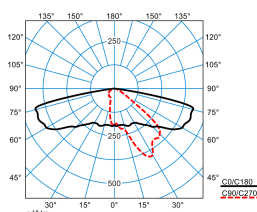
9301K AB2L-LR-SLR2/2900-730 4G3 ET (CLO end value)
