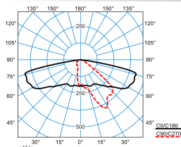
9301K AB2L-LR-SLR2/2900-730 4G3 ET (CLO initial value)
