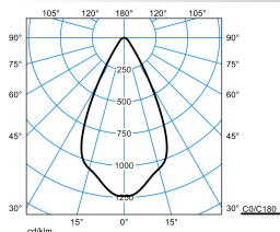
LnStar 40-RB2L/2200-740 4G1S ET
