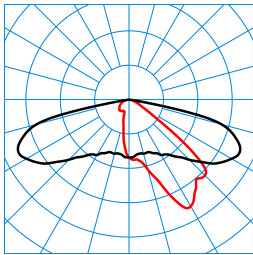
Publisca P3-AB2L-LR/6800-730 6G1 ET (CLO end value) TX301677
