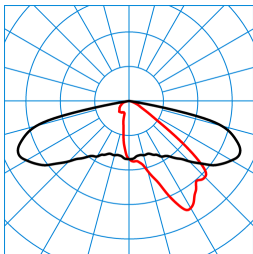
Publisca P3-AB2L-LR/6800-730 6G1 ET (CLO initial value) TX300537
