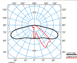
Publisca P2-AB2L/1650-740 2G1S TX047705 DIN 5040: A30 UTE: 1,00 G DLOR: 100 % ULOR: 0 % CEN Flux Code: 34 70 96 100 100
