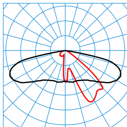
Publisca P2-AB2L/1650-740 2G1S ETDD (CLO end value) TX301691 ■ C0 - C180 ■ C90 - C270 DIN 5040: A30 UTE: 1,00 G DLOR: 100 % ULOR: 0 % CEN Flux Code: 34 70 96 100 100
