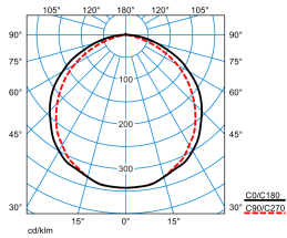
Kratex HE 600 20-840 ET Glass EB3 TX263539
